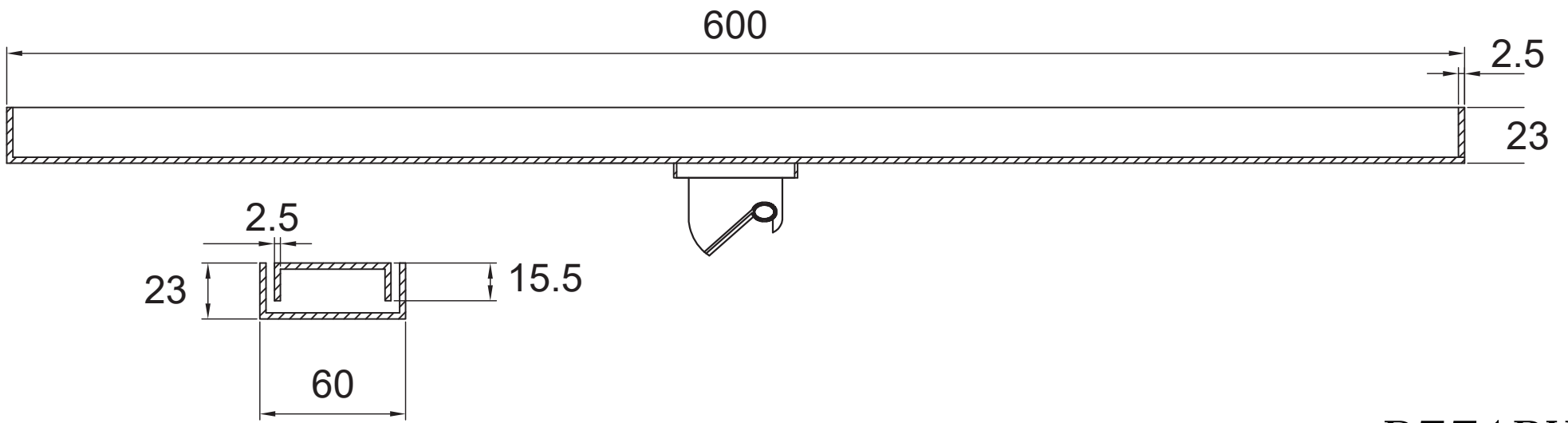
P771BH5 60*600蝶阀
