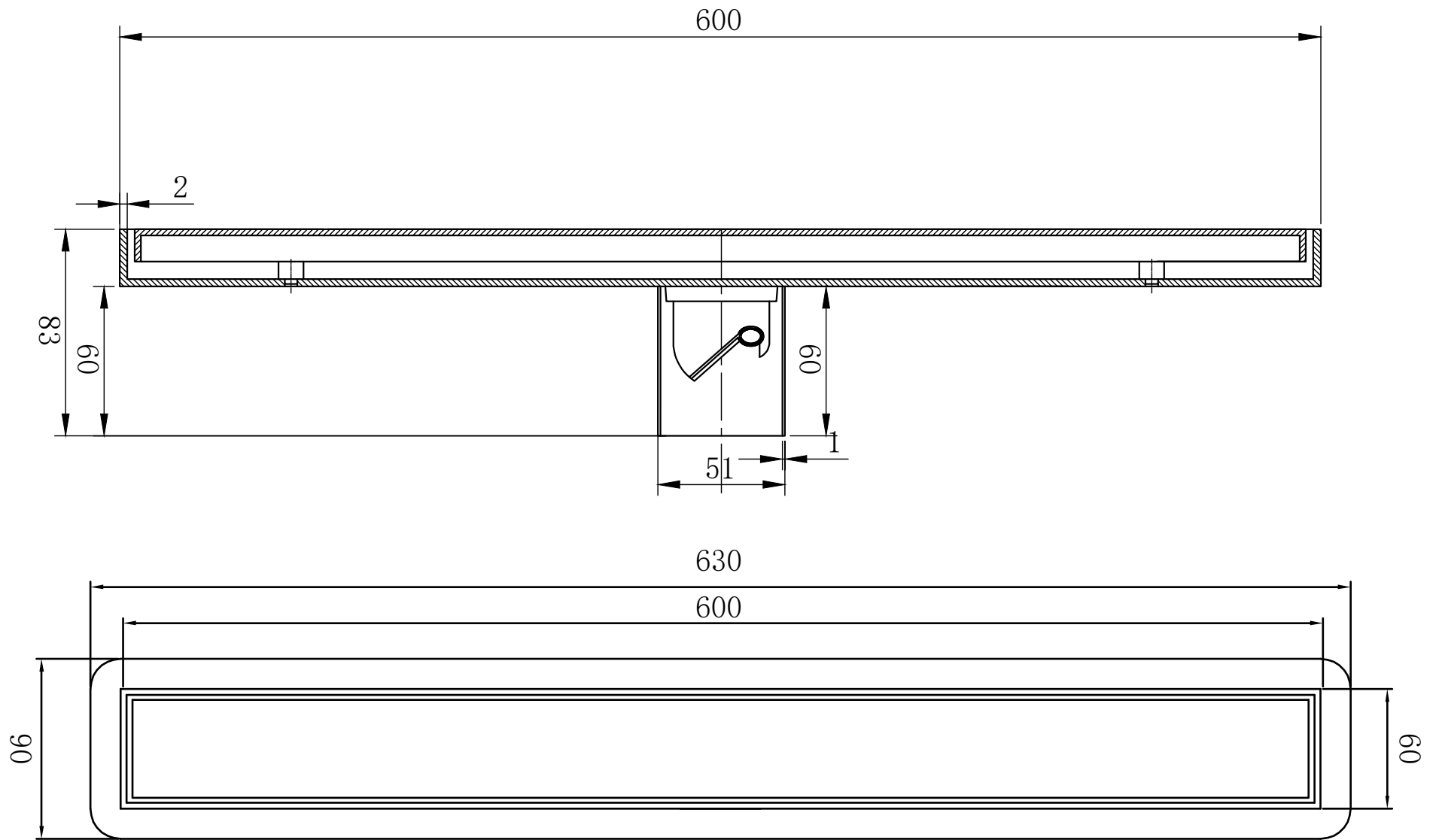
DEP778S-1 60*600蝶阀+挡水边+下水管
